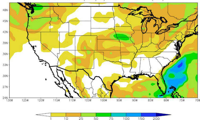
PERSPECTIVA DEL 4 AL 10 DE SEPTIEMBRE DE 2024 PRECIPITACION (mm) S/Escala – NIEVE (Viol)
